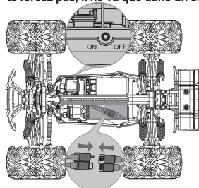
Interrupteur (Figure7)
